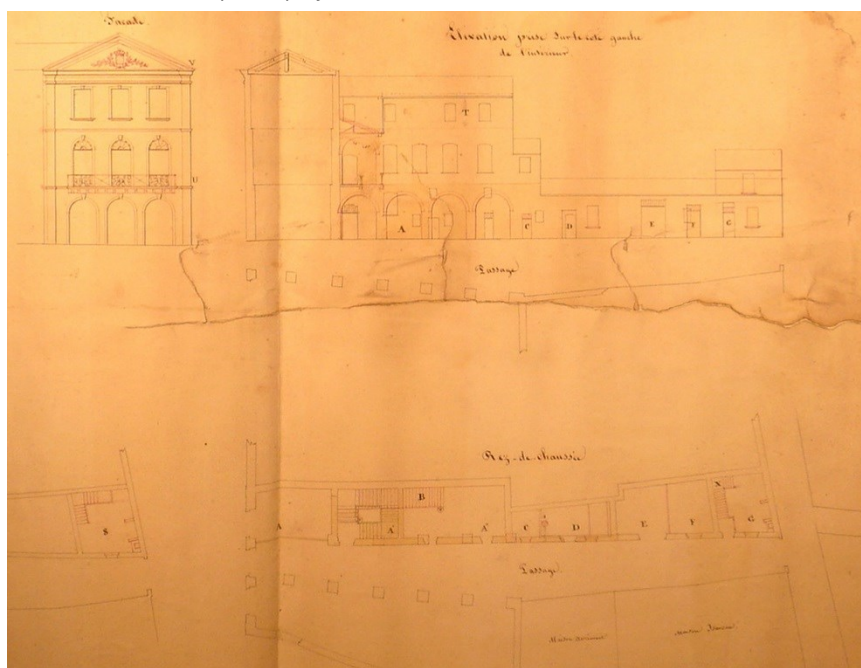
Plans, élévations, coupe du projet de restauration de l'hôtel de la mairie de Moissac. 1843. CC 57 A.M. Moissac
