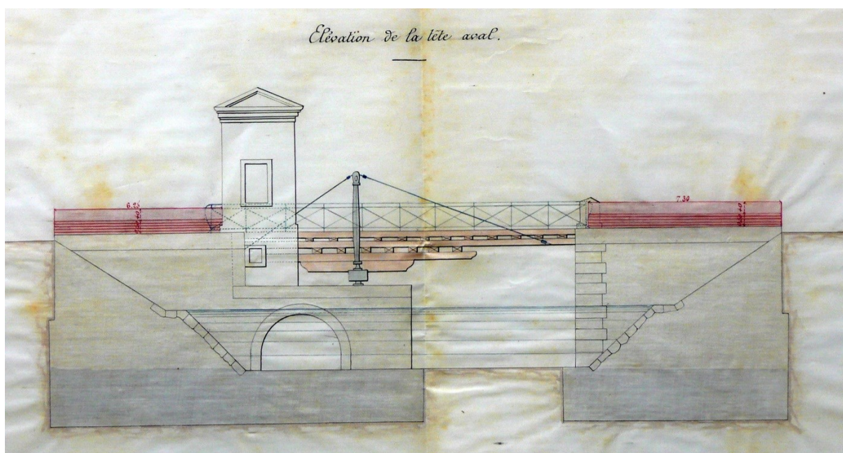
Plans, coupes, élévations - 1892. Canal latéral Parapets demandés par le conseil municipal de Moissac aux ponts tournants des Marronniers et de St Martin. Par l'ingénieur en chef des ponts et chaussées, Cie des chemins de fer du midi et du canal latéral à la Garonne. 3 O 7 A.M. Moissac
