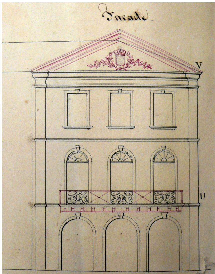
Plans, élévations, coupe du projet de restauration de l'hôtel de la mairie de Moissac.
