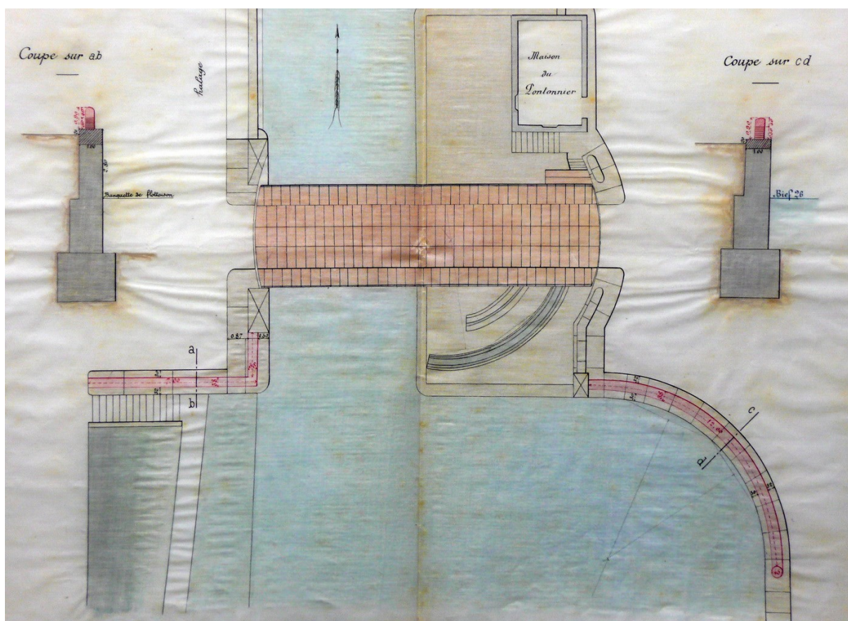
Plans, coupes, élévations - 1892. Canal latéral Parapets demandés par le conseil municipal de Moissac aux ponts tournants des Marronniers et de St Martin. Par l'ingénieur en chef des ponts et chaussées, Cie des chemins de fer du midi et du canal latéral à la Garonne. 3 O 7 A.M. Moissac
